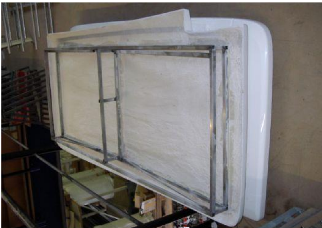
Forma spoileru - Forma vyrobená z Acrystal Prima s epoxidovým gelcoatem – Fiberfab - Ilsfeld - Německo
